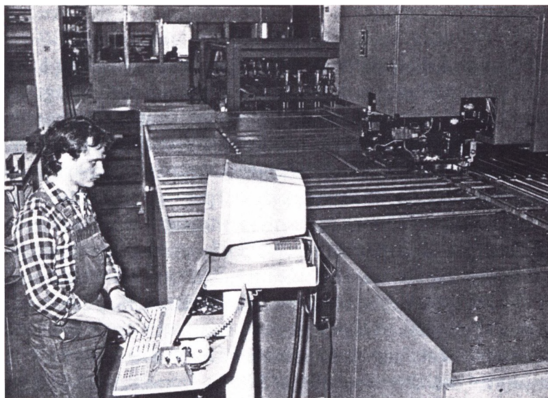
Fra Nyborg Vaskerimaskiner. Datamatstyret stanse- og klippecenter.
